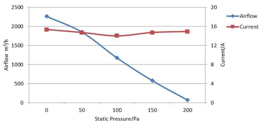
305mm 有刷轴流风机 12V DC 305mm Brush Axial Fan
