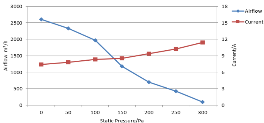
305mm 有刷轴流风机 24V DC 305mm Brush Axial Fan
