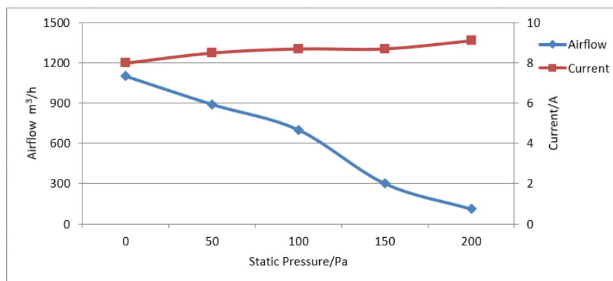
225mm 有刷轴流风机 12V DC 225mm Brushed Axial Fan
